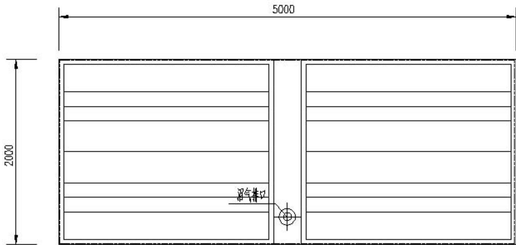
方形池三相分离器平面图大样
