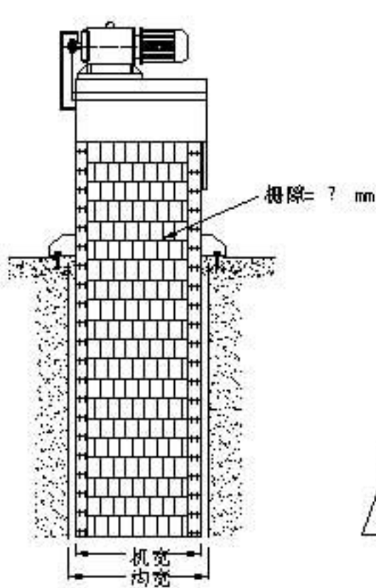
格栅正面图
