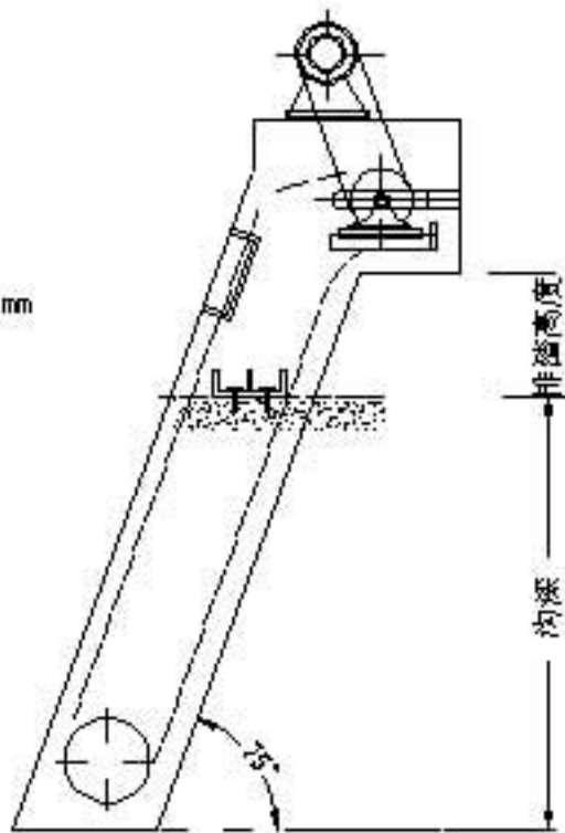
格栅侧面图
